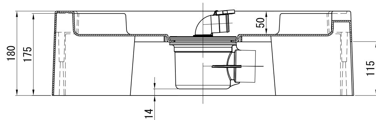
断面 A-A
